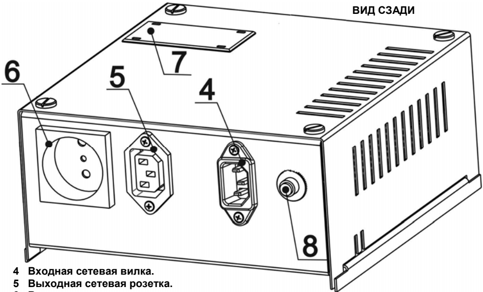
Рис.1 Расположение органов управления, коммутации и индикации.
