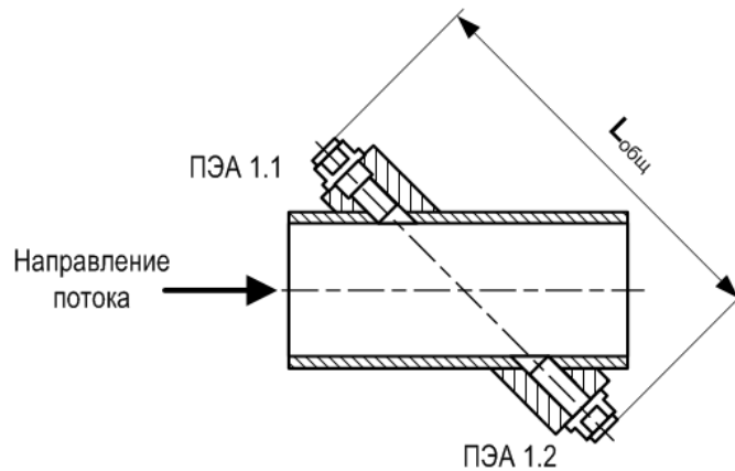
Рис.10. Измеряемое расстояние между парой ПЭА.
