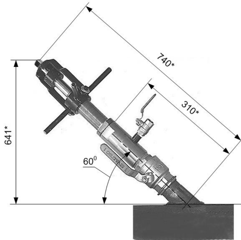
Рис.А.5. Комплект монтажный «ВЗЛЕТ КПВД» в рабочем положении.
