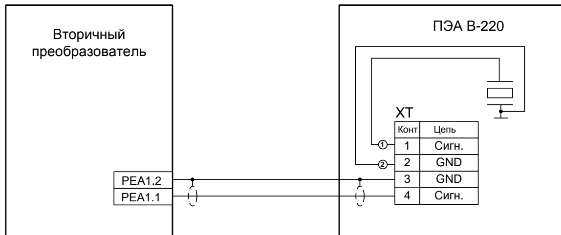
Рис.Б.1. Схема подключения пары ПЭА В-220.
