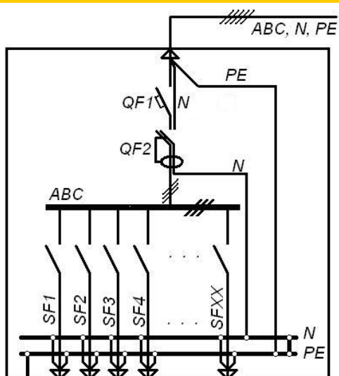
Рис.17.8 ЩРН(В)1-3-XXX-XXXX-XXУХЛ4-X
