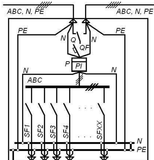
Рис.17.11 ЩУРН(В)2-3-XXX-XXXX-XXУХЛ4
