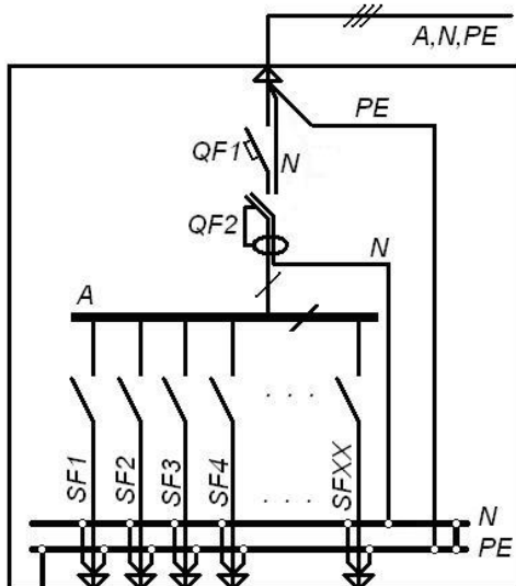
Рис.17.4 ЩРН(В)1-1-XXX-00XX-XXУХЛ4-X
