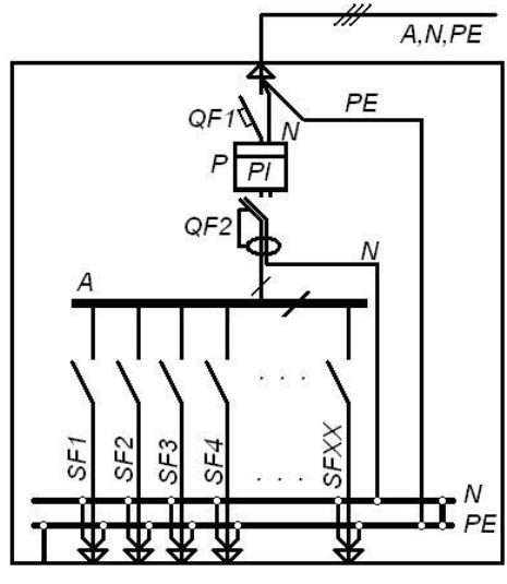
Рис.17.5. ЩУРН(В)1-1-XXX-00XX-XXУХЛ4-X
