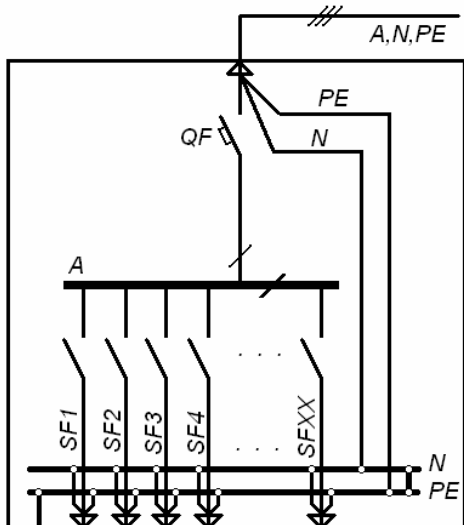
Рис.17.2 ЩРН(В)1-1-XXX-00XX-XXУХЛ4
