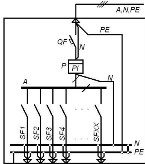
Рис.17.3 ЩУРН(В)1-1-XXX-00XX-XXУХЛ4
