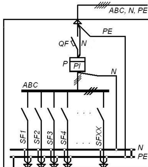
Рис.17.7 ЩУРН(В)1-3-XXX-XXXX-XXУХЛ4
