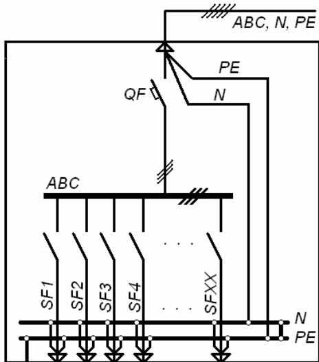
Рис.17.6 ЩРН(В)1-3-XXX-XXXX-XXУХЛ4
