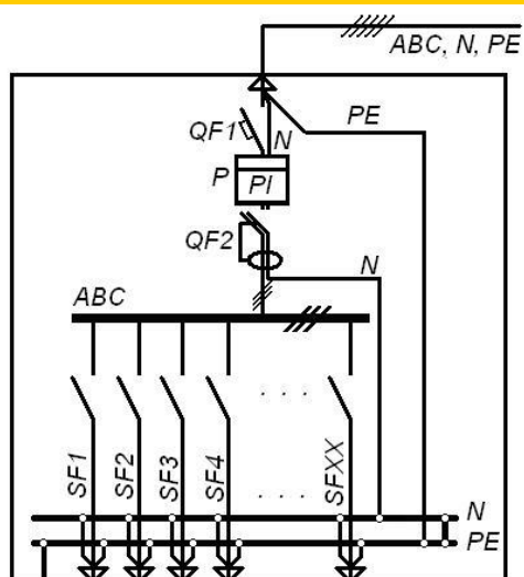
Рис.17.9 ЩУРН(В)1-3-XXX-XXXX-XXУХЛ4-X
