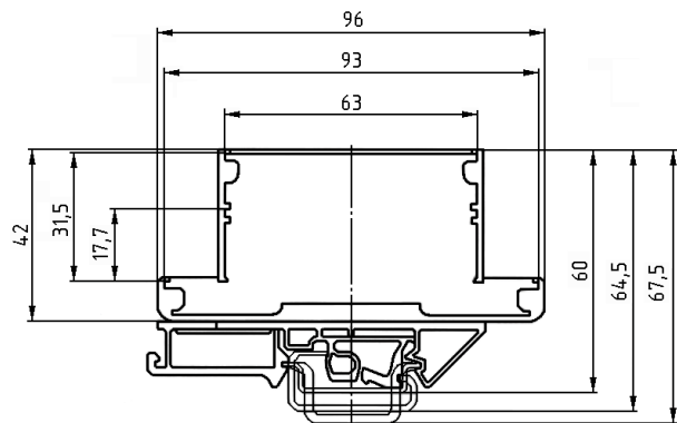
б) в открытом корпусе с универсальным креплением для монтажа на DIN рейку 32/35. Рисунок 2. Габаритные размеры устройства управления оповещателем YVO-RGB.
