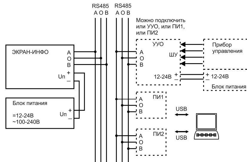
Рисунок 3. Схема соединений YVO-RGB и ЭКРАН-ИНФО-RGB.
