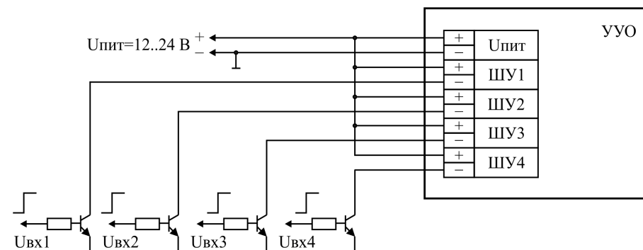
Рисунок 4. Схема каскада входа управления ШУ YVO-RGB
