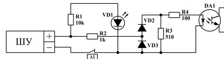
Рисунок 4. Схема каскада входа управления ШУ YVO-RGB
